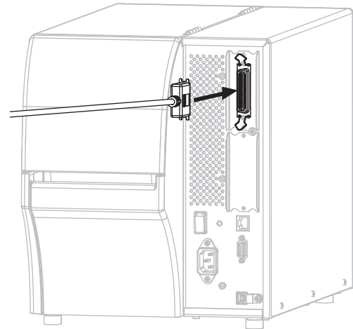
Connecteur parallèle
