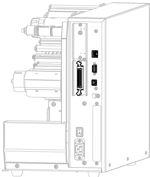
Figure18 Emplacement des interfaces de communication
