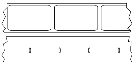
Espace/encoche
