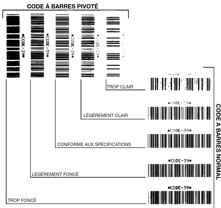
Figure 3 Comparaison des contrastes des codes à barres
