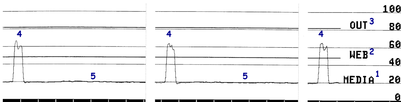
Figure 7 Profil de cellule papier (papier à espace/encoche)
