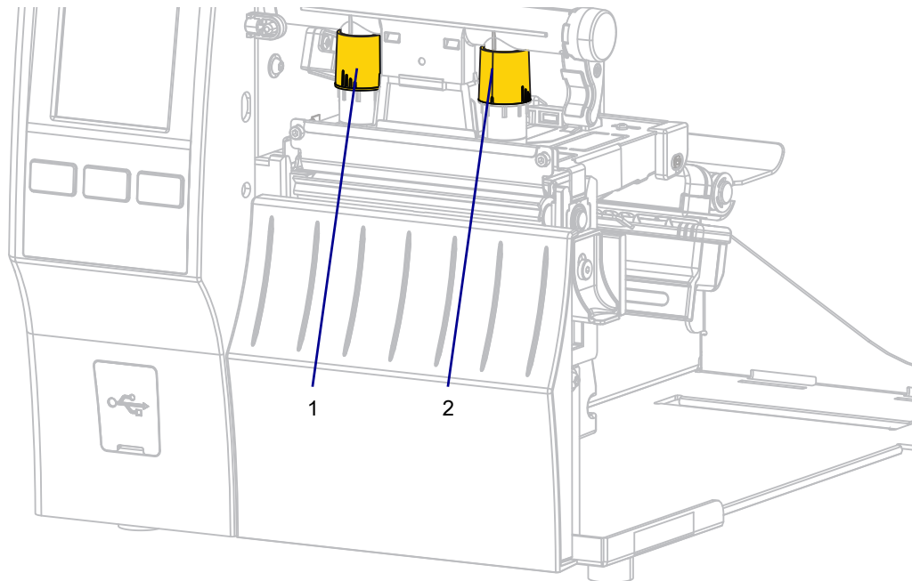
Figure 2 Cadrans de réglage de pression de la tête
