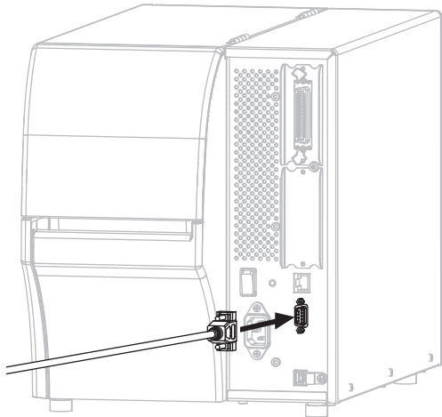
Connecteur série
