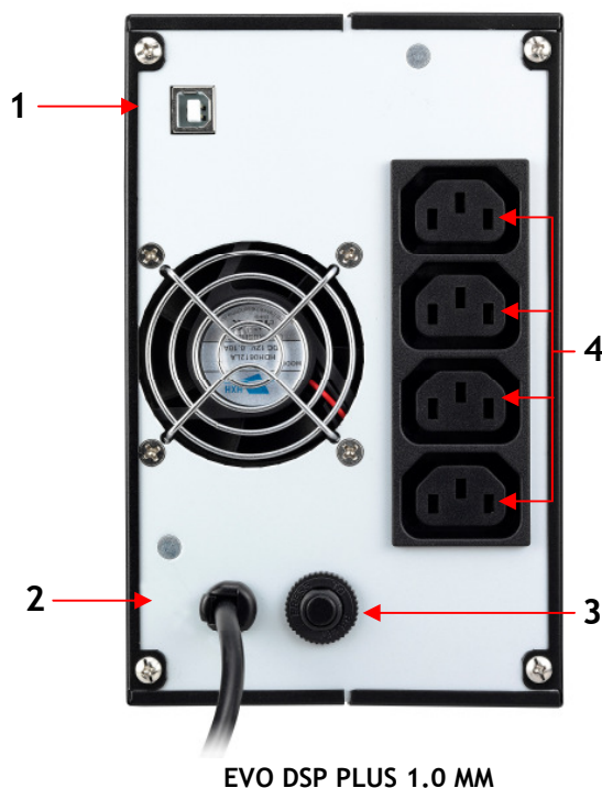
Figura 4 - Pannello Posteriore
