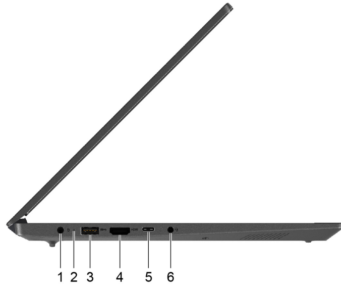
Figura 7. Vista laterale sinistra—modelli da 15 pollici
