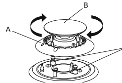
Рис. 10: позиционирование конфорок серии III
