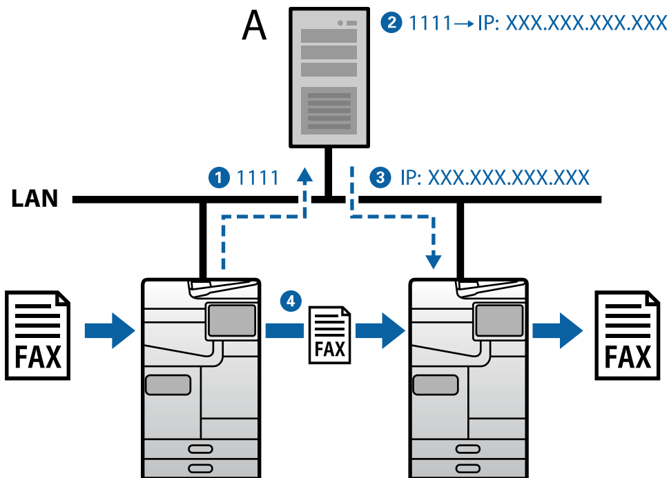
A: SIP Server
