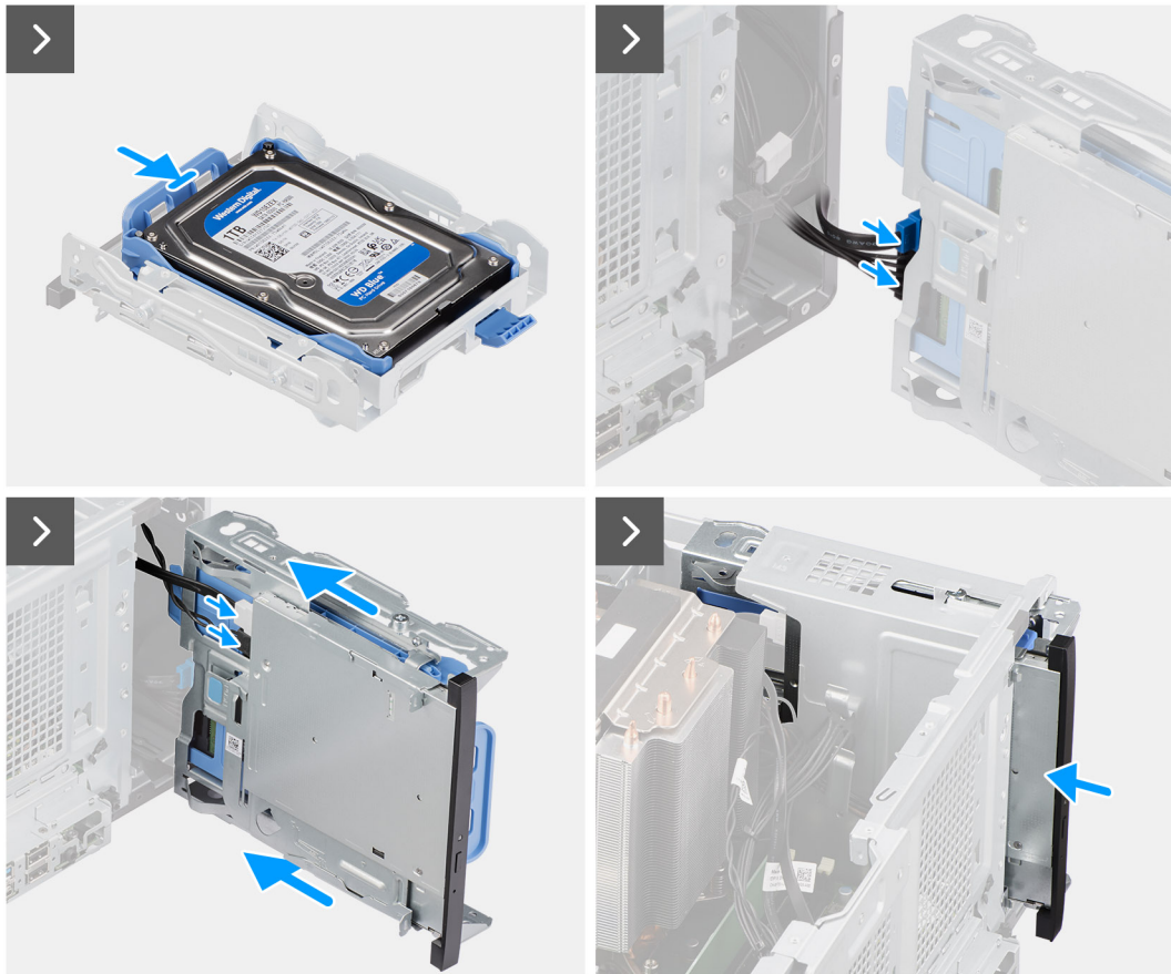
Figura 38. Installazione del disco rigido da 3,5 pollici
