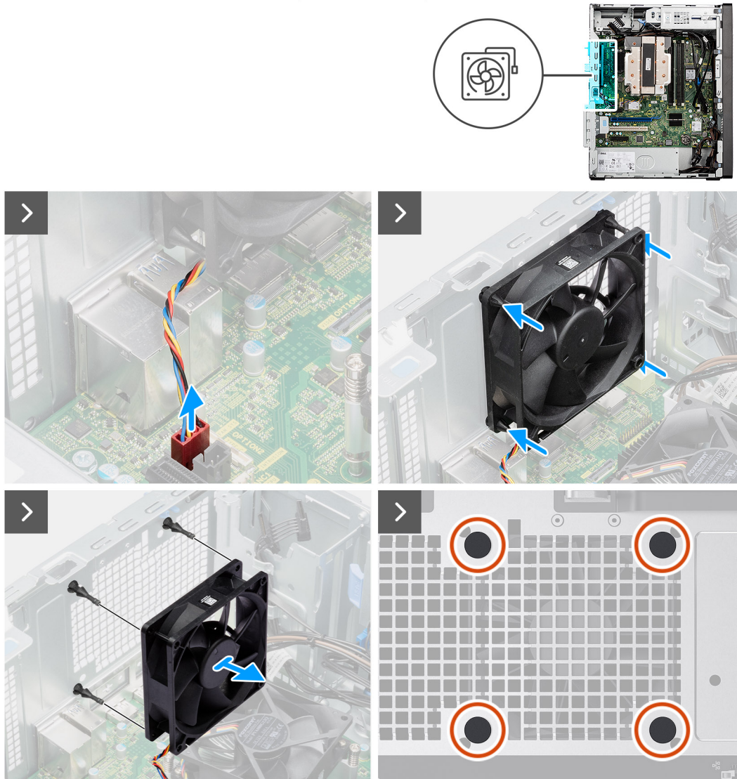
Figura 78. Rimozione della ventola di sistema
