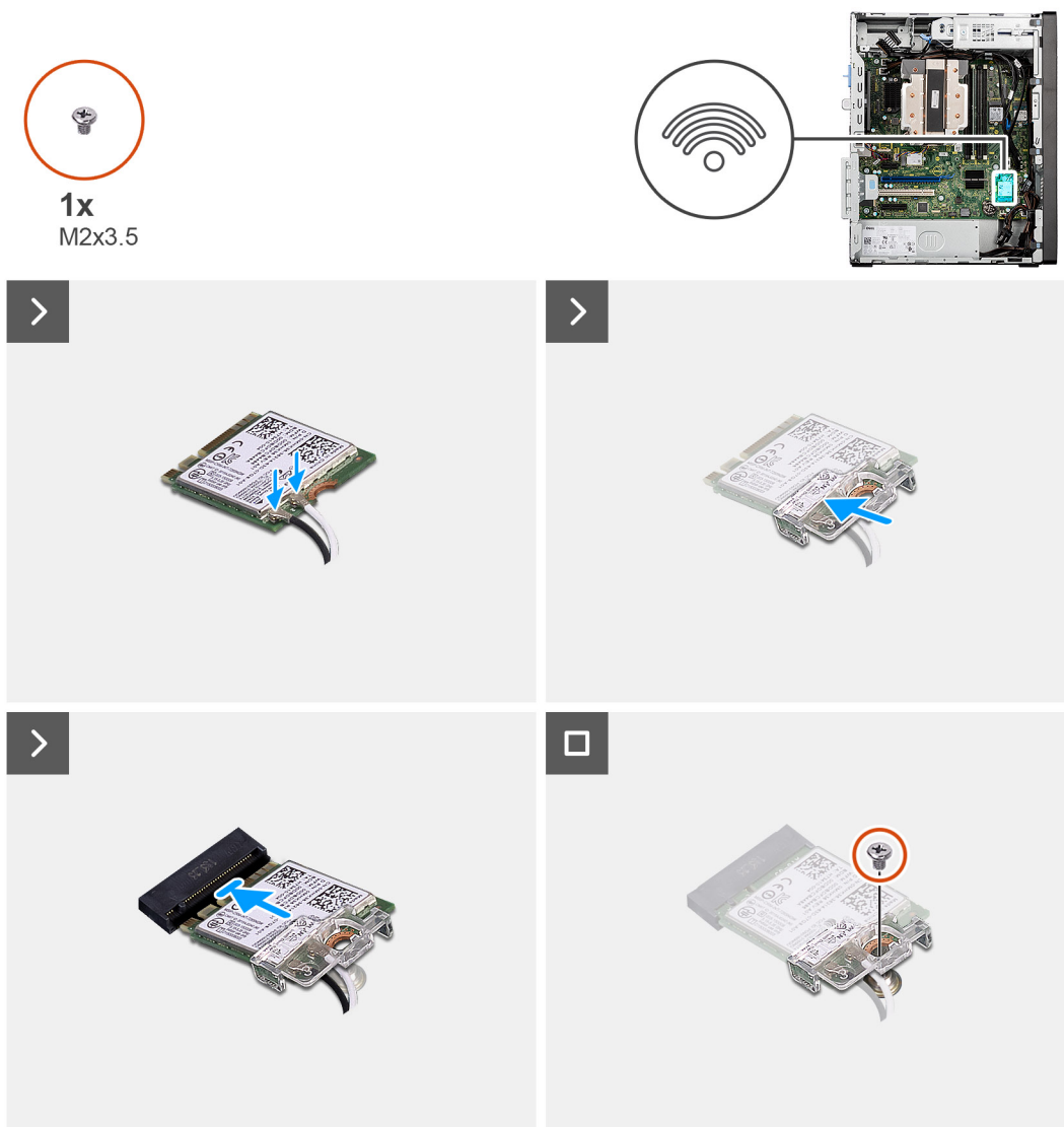
Figura 25. Installazione della scheda wireless
