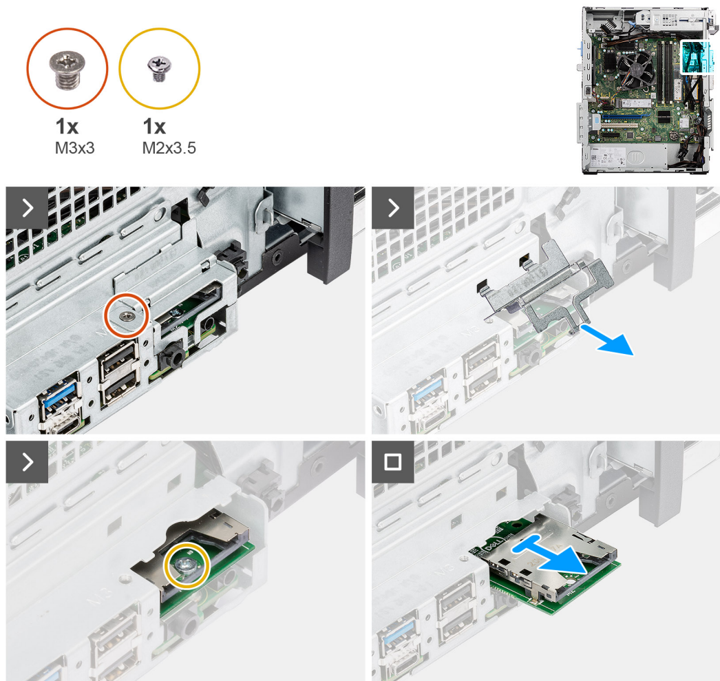
Figura 32. Rimozione del lettore di schede multimediali
