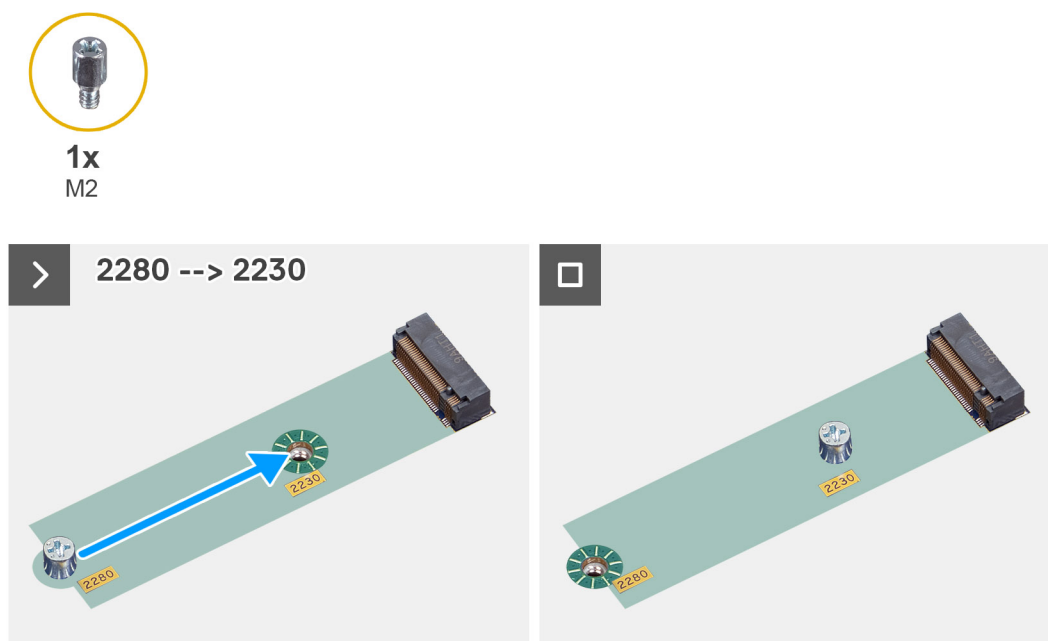
Figura 19. Installazione dell'unità SSD M.2 2230
