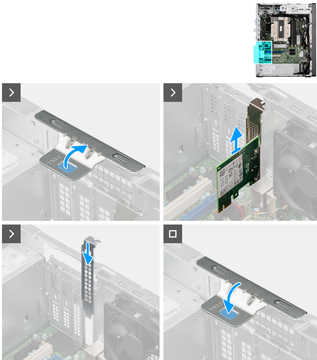
Figura 52. Rimozione della scheda di rete
