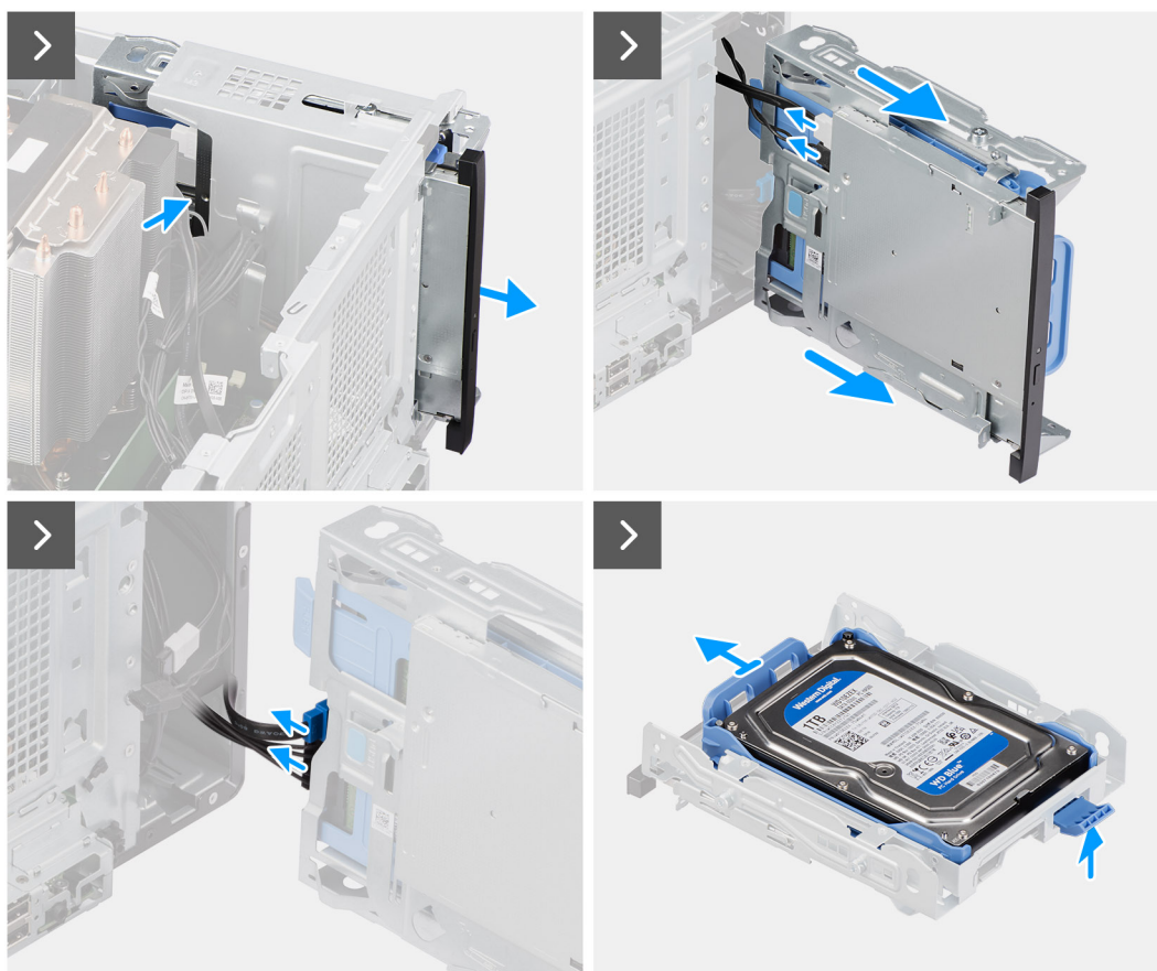
Figura 35. Rimozione del disco rigido da 3,5 pollici
