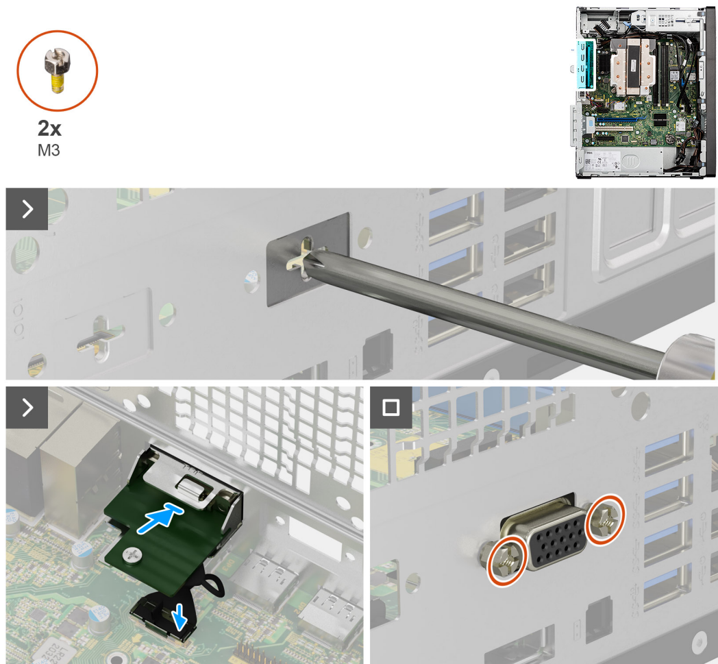
Figura 93. Installare il modulo VGA opzionale.
