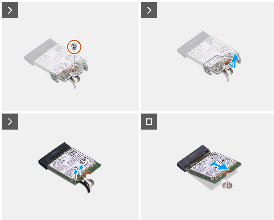
Figura 24. Rimozione della scheda wireless
