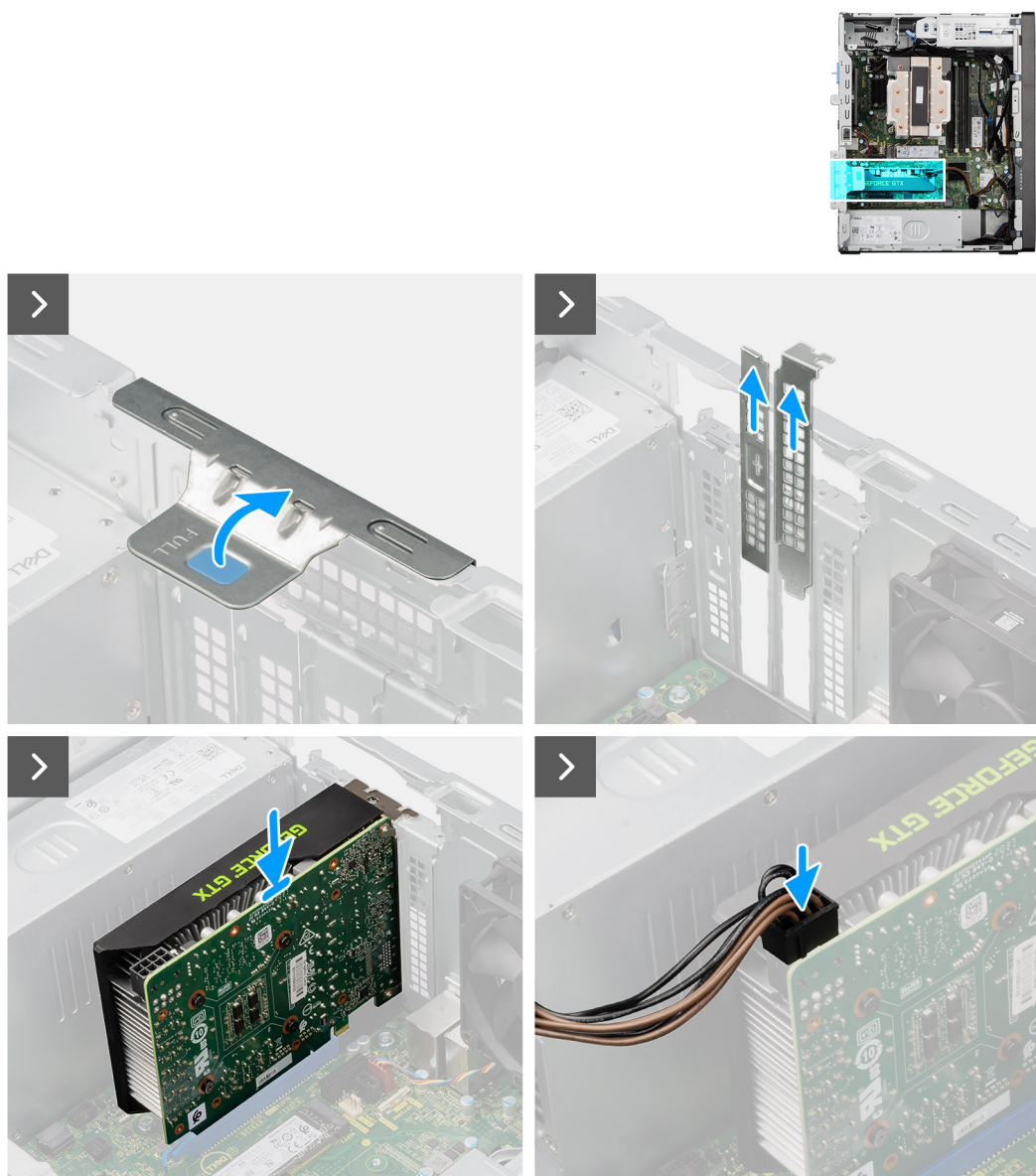
Figura 30. Installazione della scheda grafica alimentata
