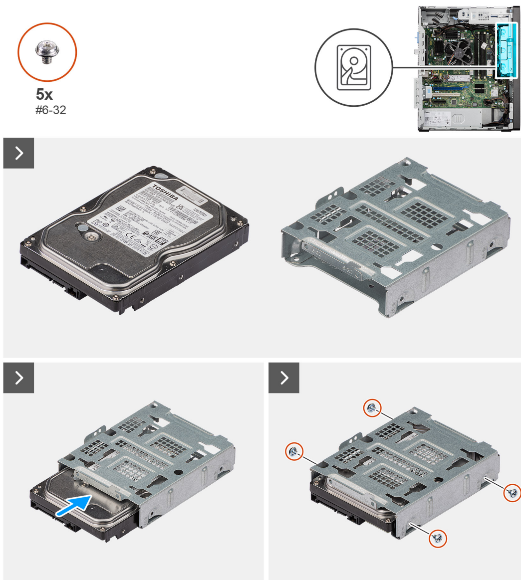
Figura 42. Installazione del disco rigido secondario da 3,5 pollici
