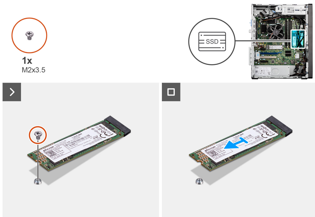
Figura 21. Rimozione dell'unità SSD M.2 2280
