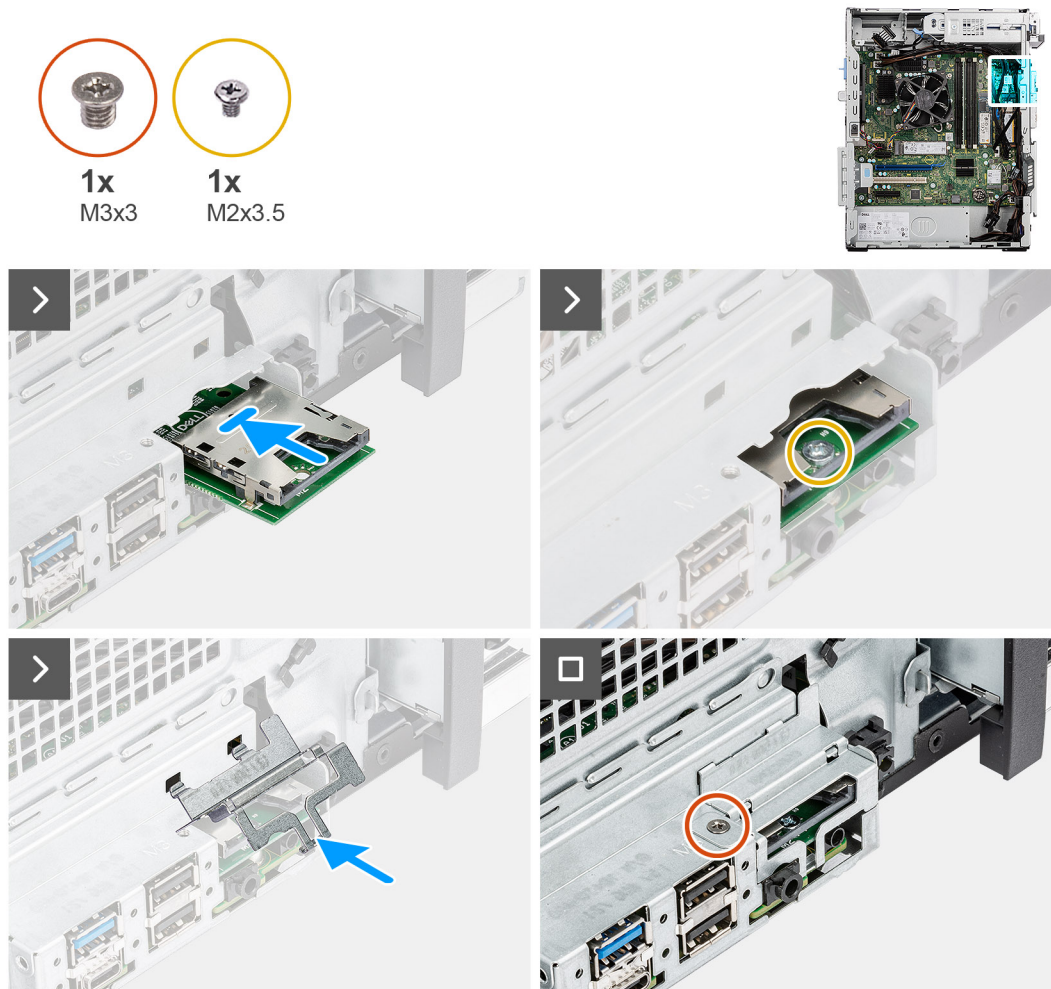
Figura 33. Installazione del lettore di schede multimediali
