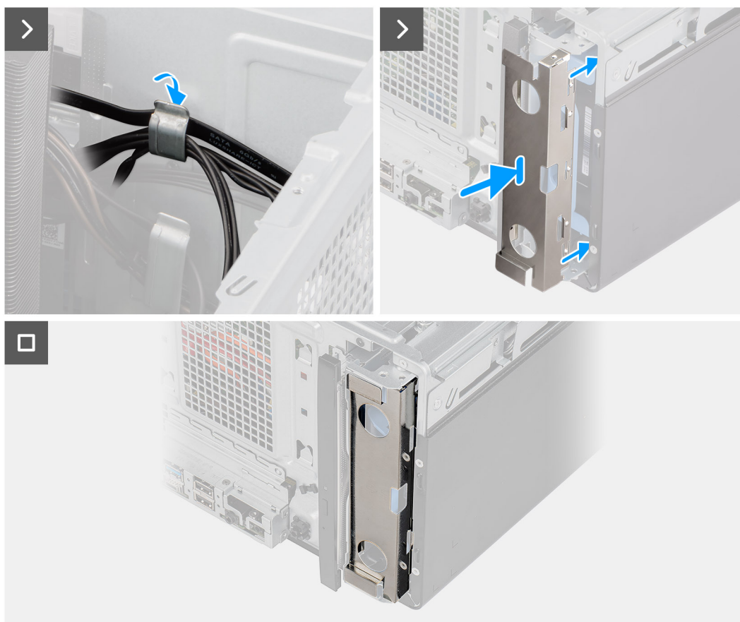
Figura 49. Installazione dell'unità ottica slim
