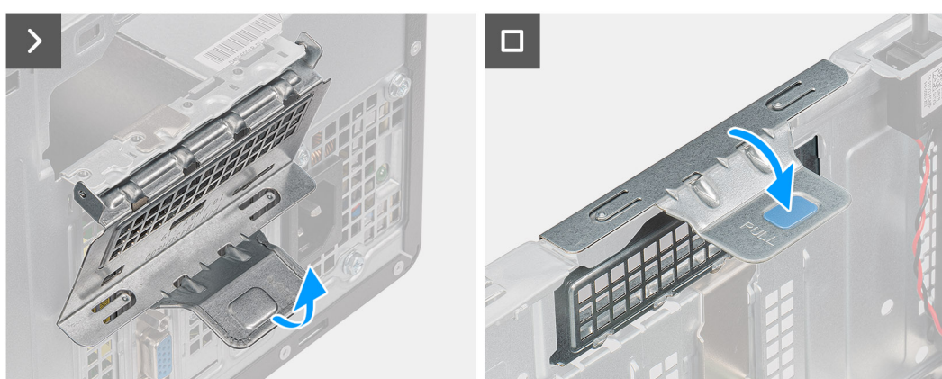
Figura 57. Rimozione della scheda delle porte seriali/parallele
