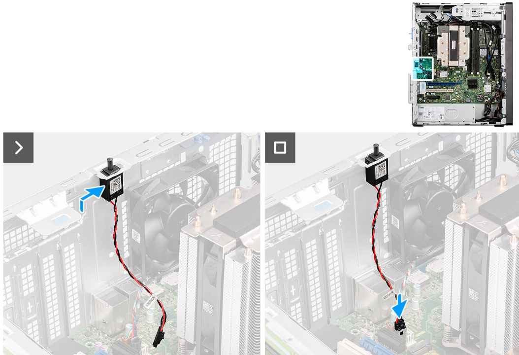
Figura 59. Installazione dell'interruttore di apertura
