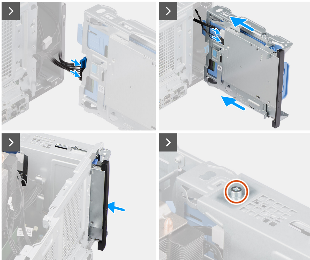
Figura 48. Installazione dell'unità ottica slim
