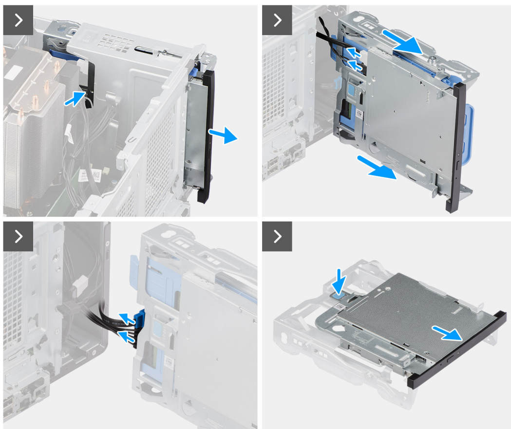
Figura 45. Rimozione dell'unità ottica slim
