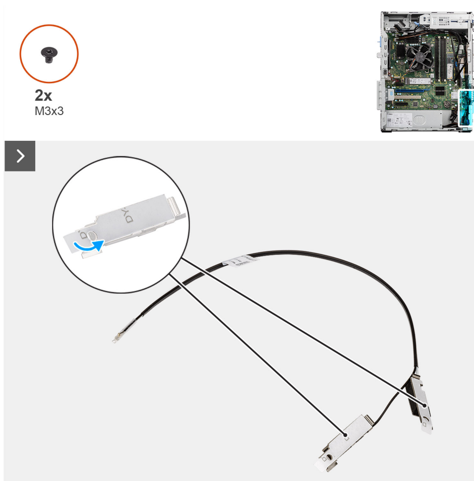
Figura 64. Installazione del modulo dell'antenna interna
