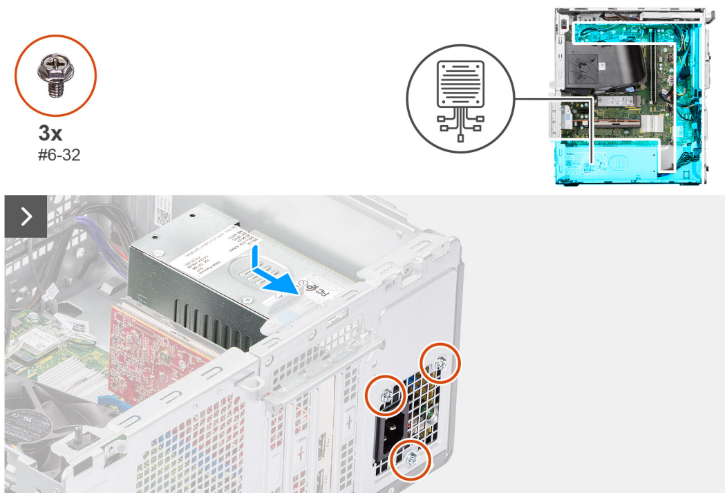
Figura 66. Installazione dell'unità di alimentazione
