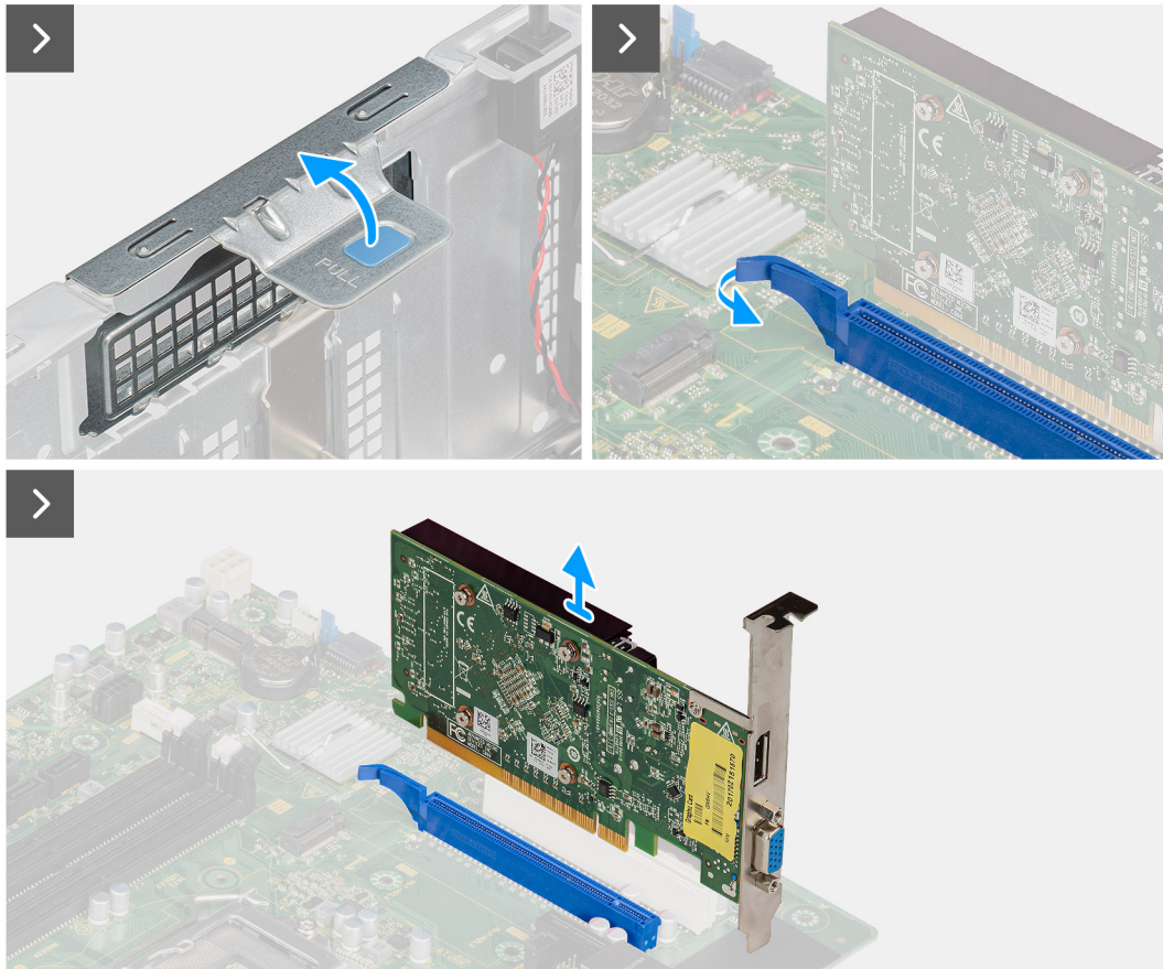
Figura 43. Rimozione della scheda delle porte seriali/parallele
