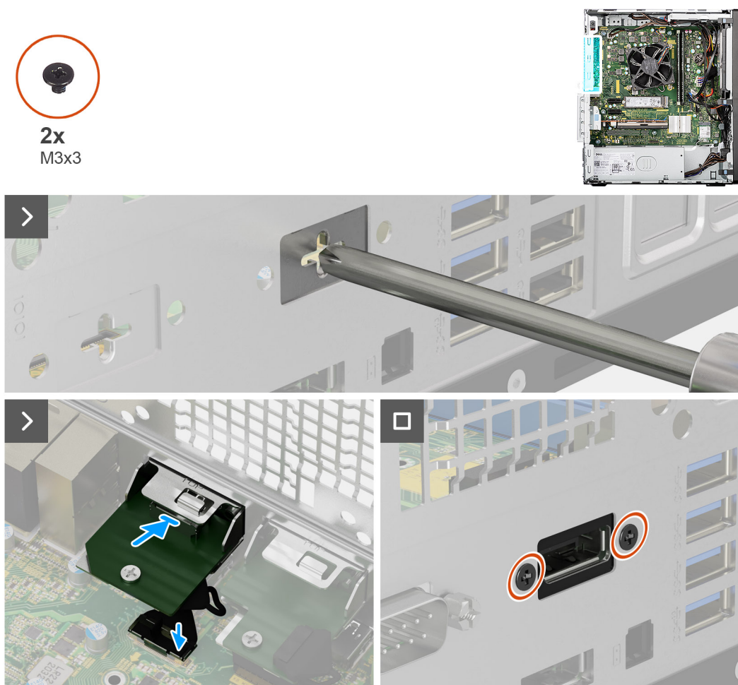
Figura 79. Installare il modulo DisplayPort opzionale.
