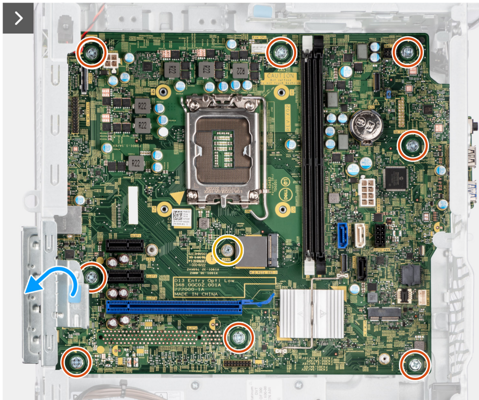
Figura 85. Rimozione della scheda di sistema
