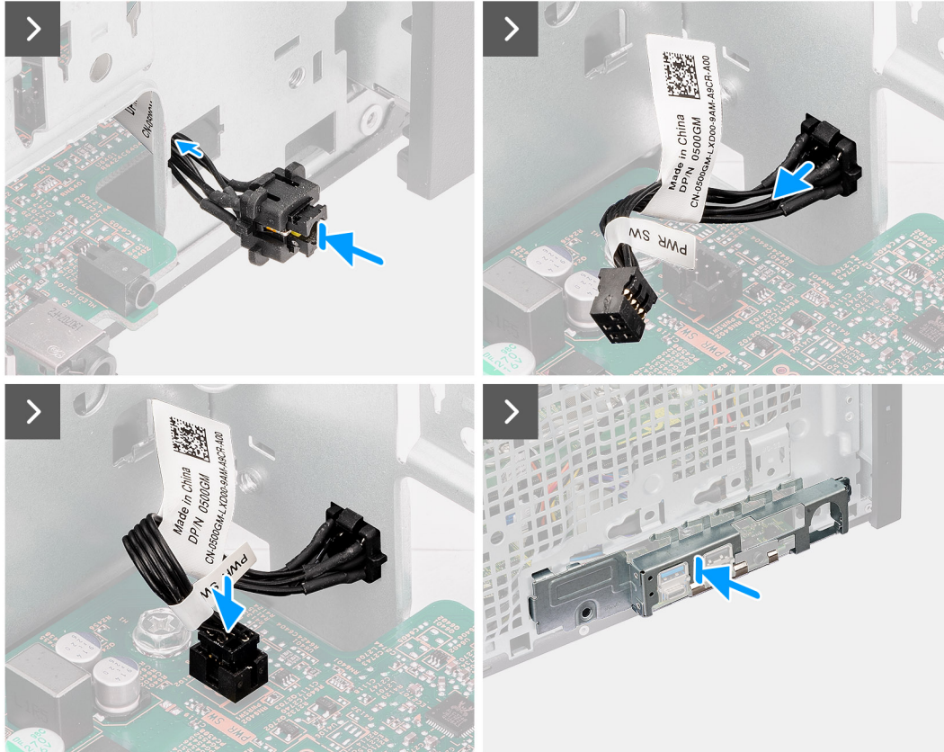
Figura 50. Installazione del pulsante di accensione
