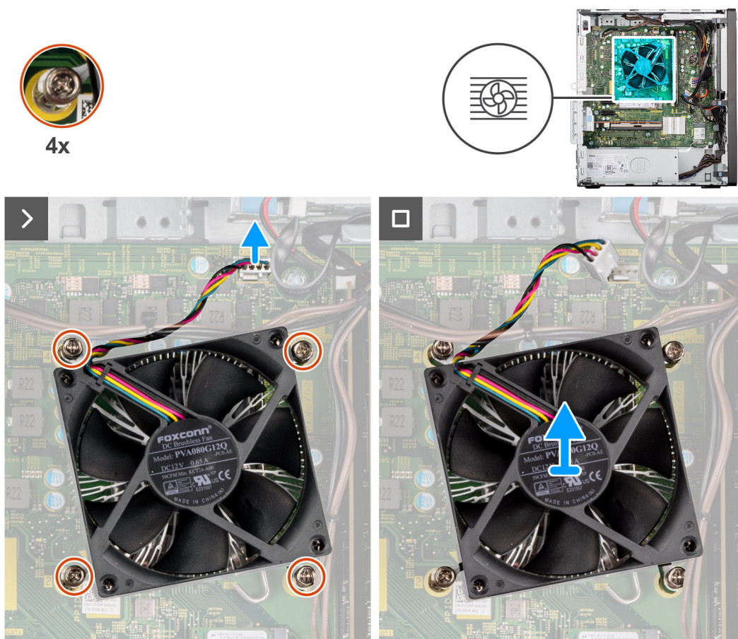
Figura 62. Rimozione del gruppo ventola del processore e dissipatore di calore
