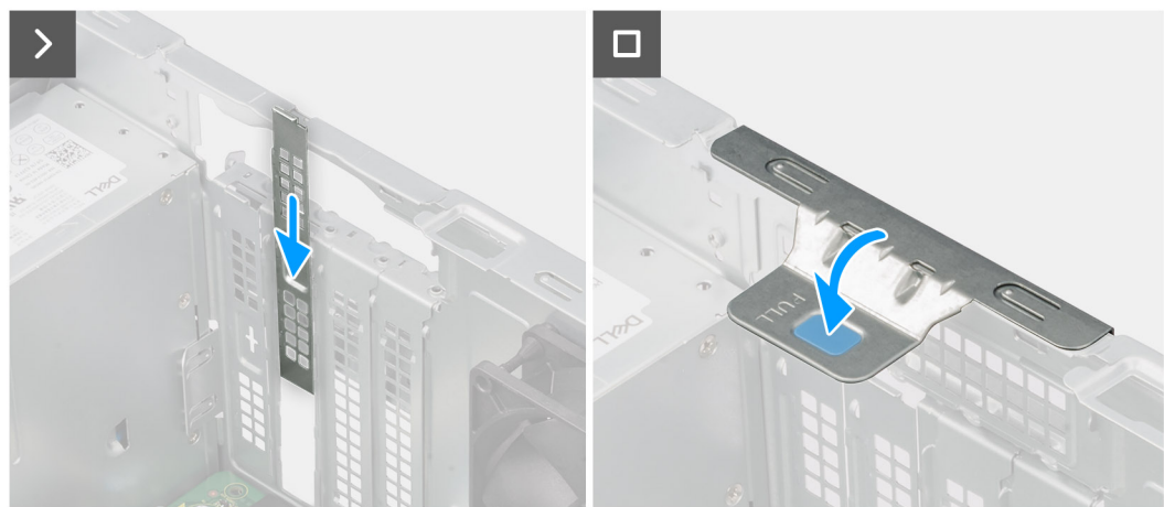
Figura 44. Rimozione della scheda delle porte seriali/parallele
