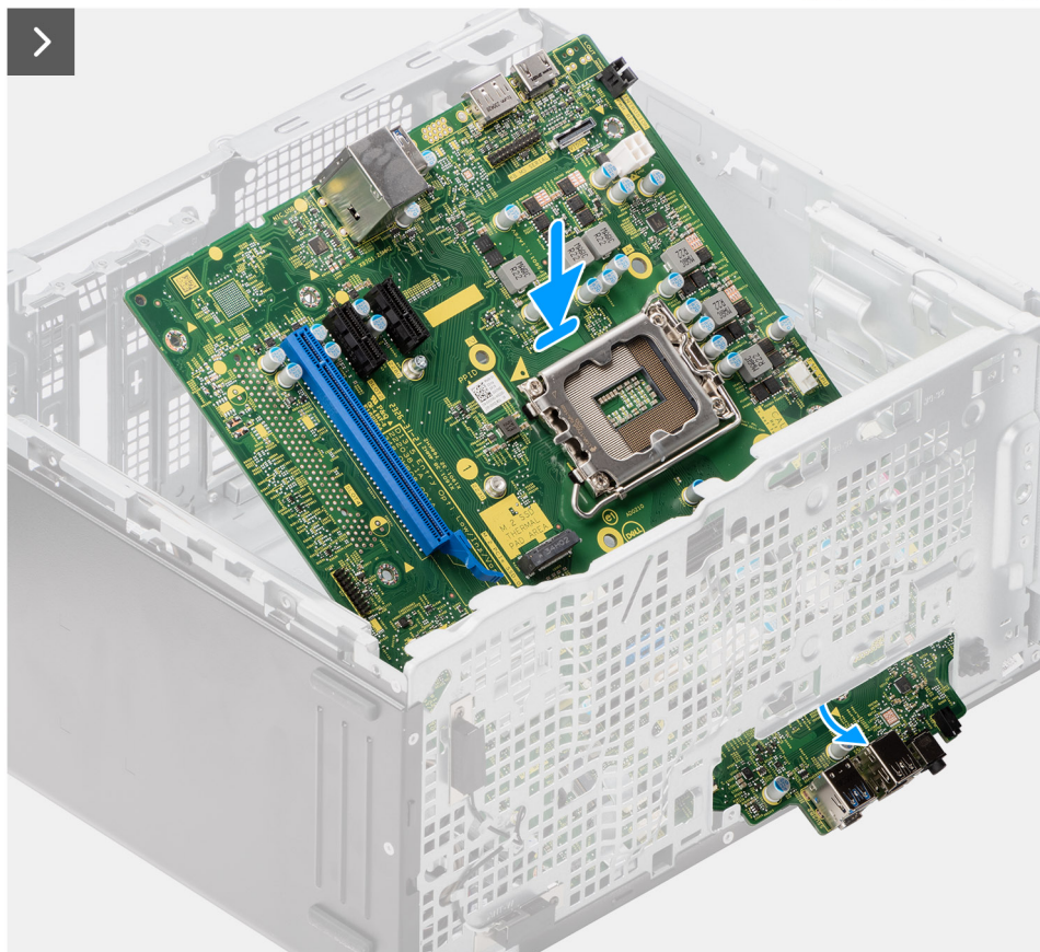
Figura 88. Installazione della scheda di sistema
