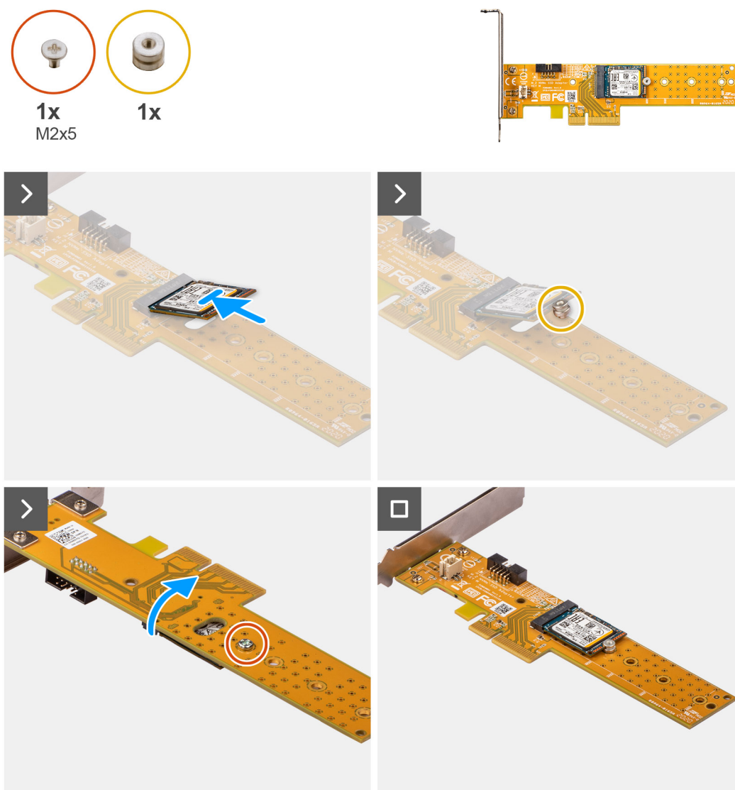
Figura 28. Installazione della scheda Dell Ultra Speed Drive Gen3 con unità SSD M.2 2230
