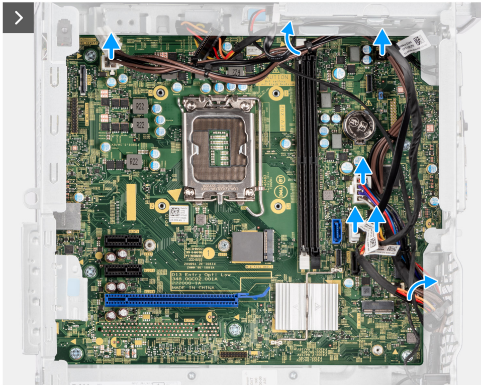
Figura 84. Rimozione della scheda di sistema
