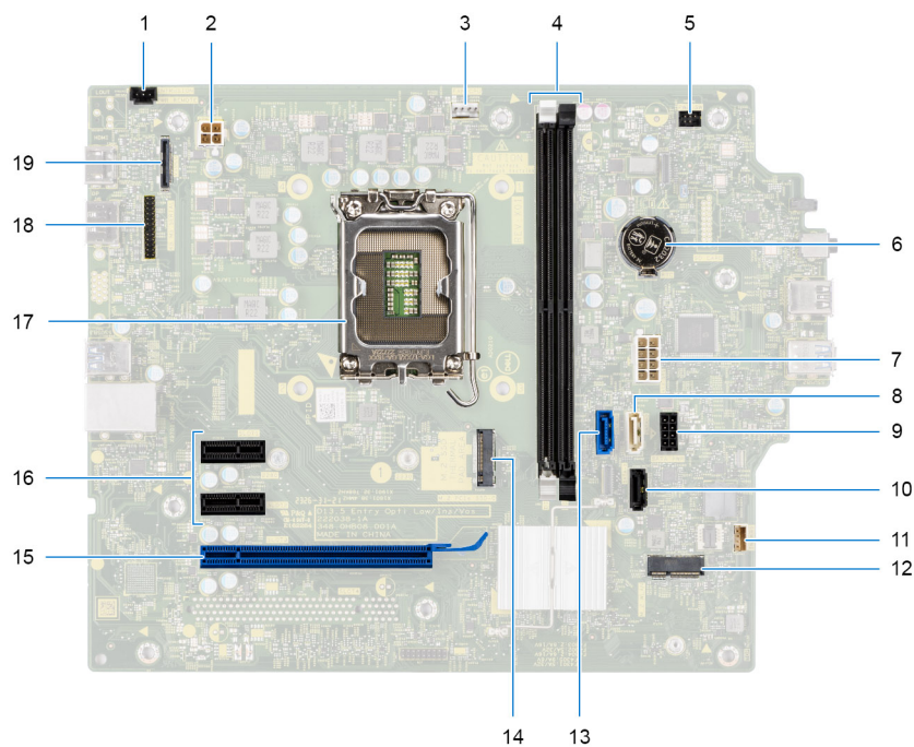
Figura 82. Connettori della scheda di sistema
