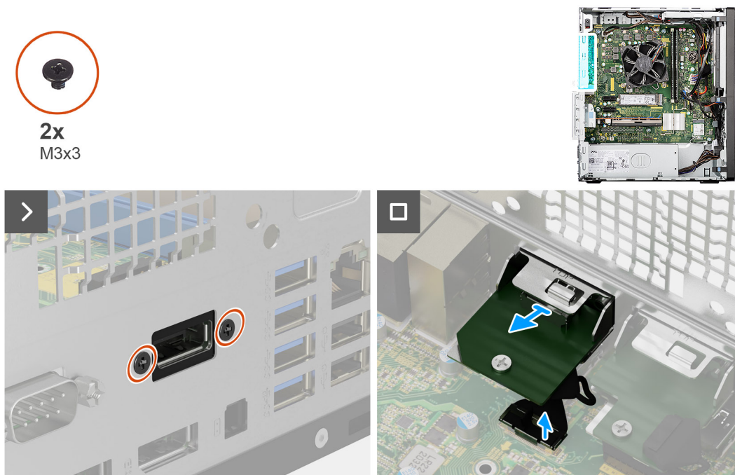
Figura 78. Rimozione del modulo DisplayPort opzionale
