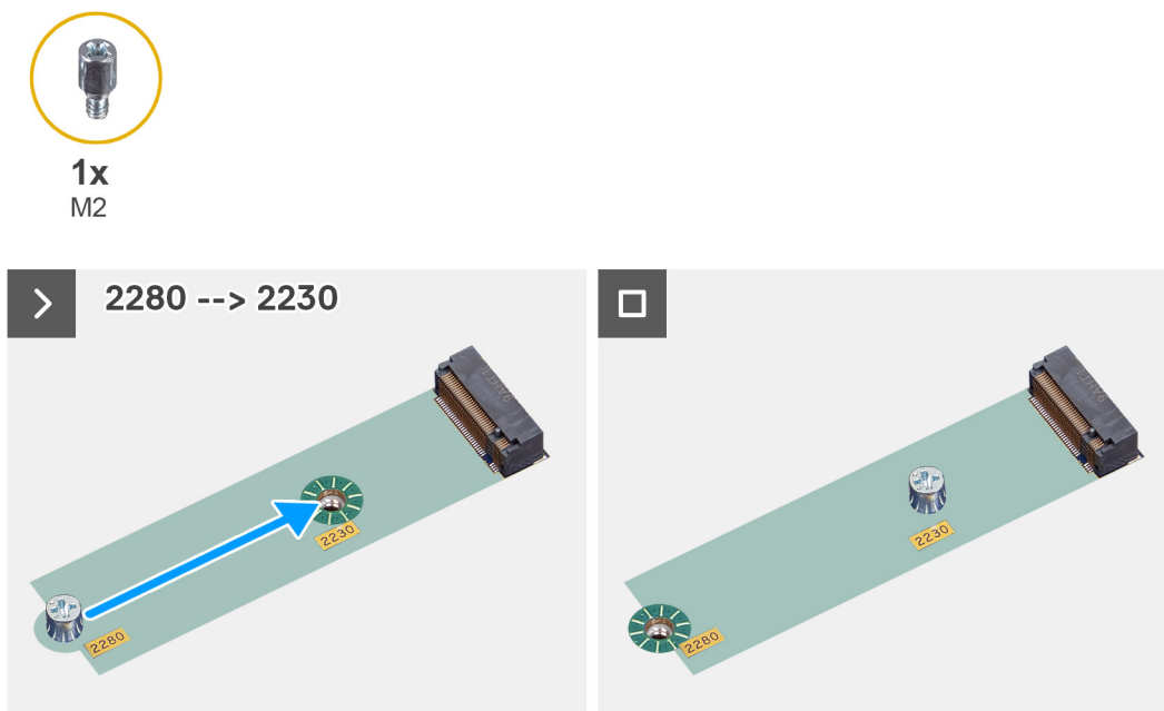
Figura 20. Installazione dell'unità SSD M.2 2230
