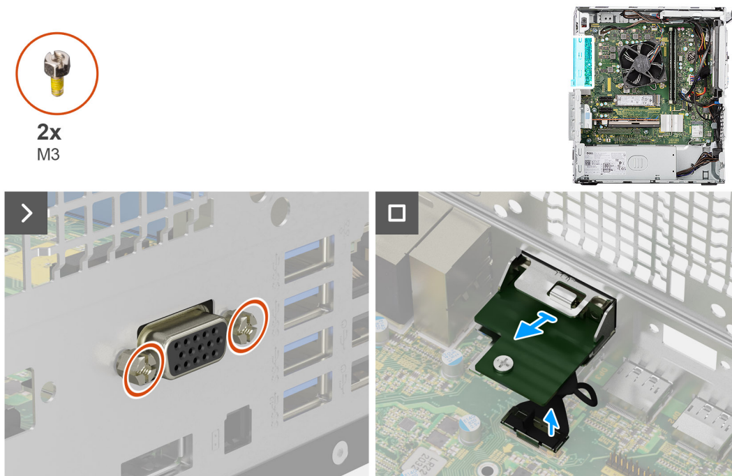
Figura 80. Rimozione del modulo VGA opzionale
