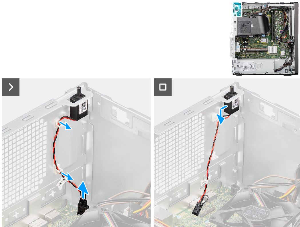
Figura 47. Rimozione dell'interruttore di intrusione
