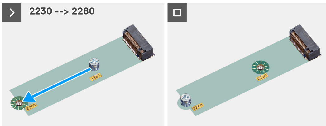
Figura 23. Installazione dell'unità SSD M.2 2230
