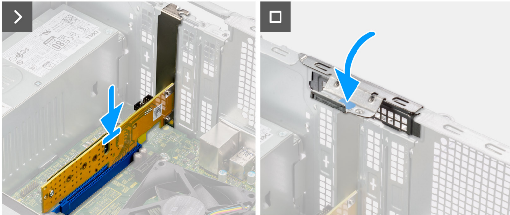
Figura 30. Installazione della scheda Dell Ultra Speed Drive Gen3
