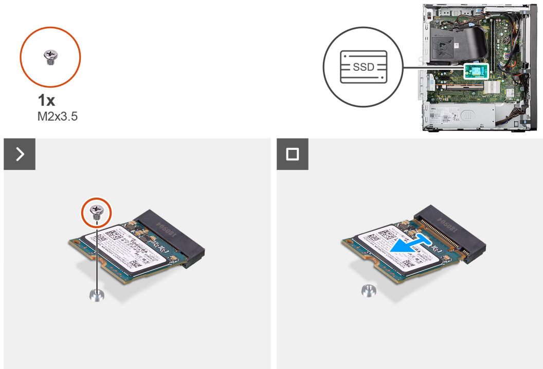
Figura 19. Rimozione dell'unità SSD M.2 2230
