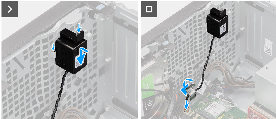
Figura 42. Installazione dell'altoparlante interno
