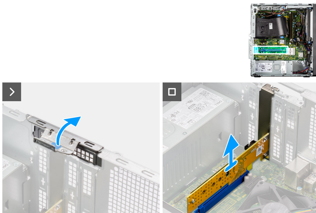
Figura 25. Rimozione della scheda Dell Ultra Speed Drive Gen3
