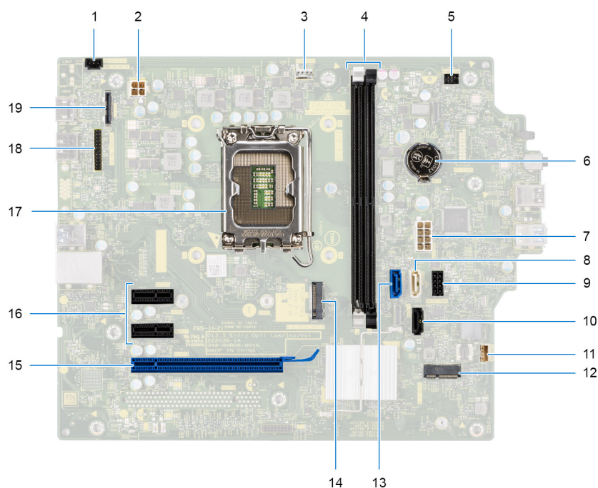
Figura 87. Connettori della scheda di sistema
