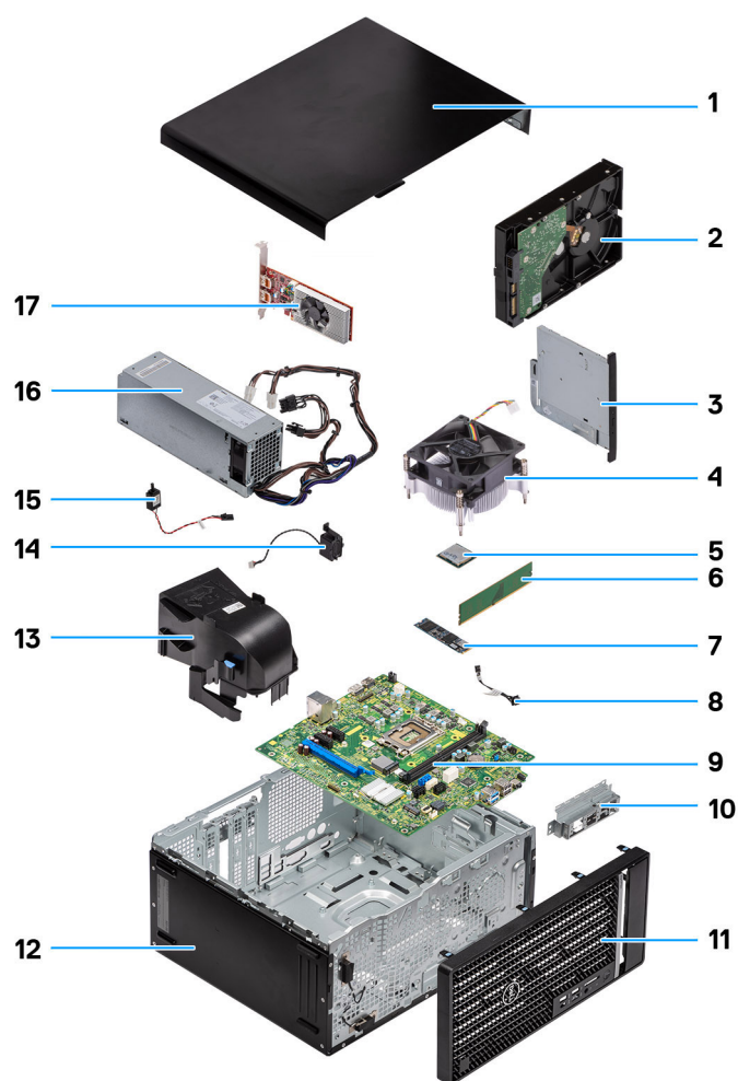
Figura 8. Componenti principali di OptiPlex Tower 7020
