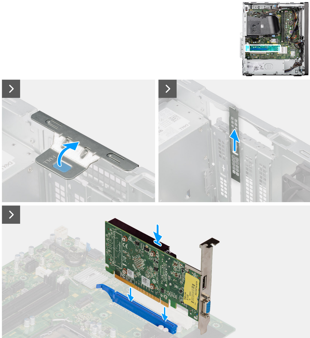
Figura 45. Installazione della scheda delle porte seriali/parallele
