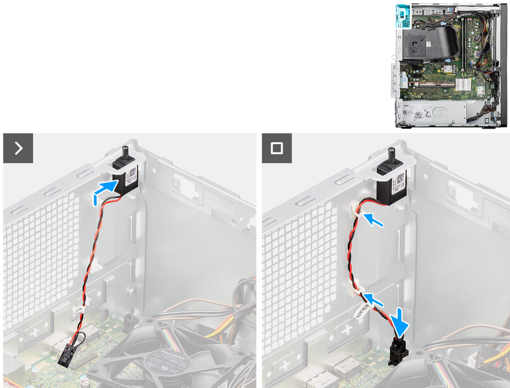
Figura 48. Installazione dell'interruttore di apertura
