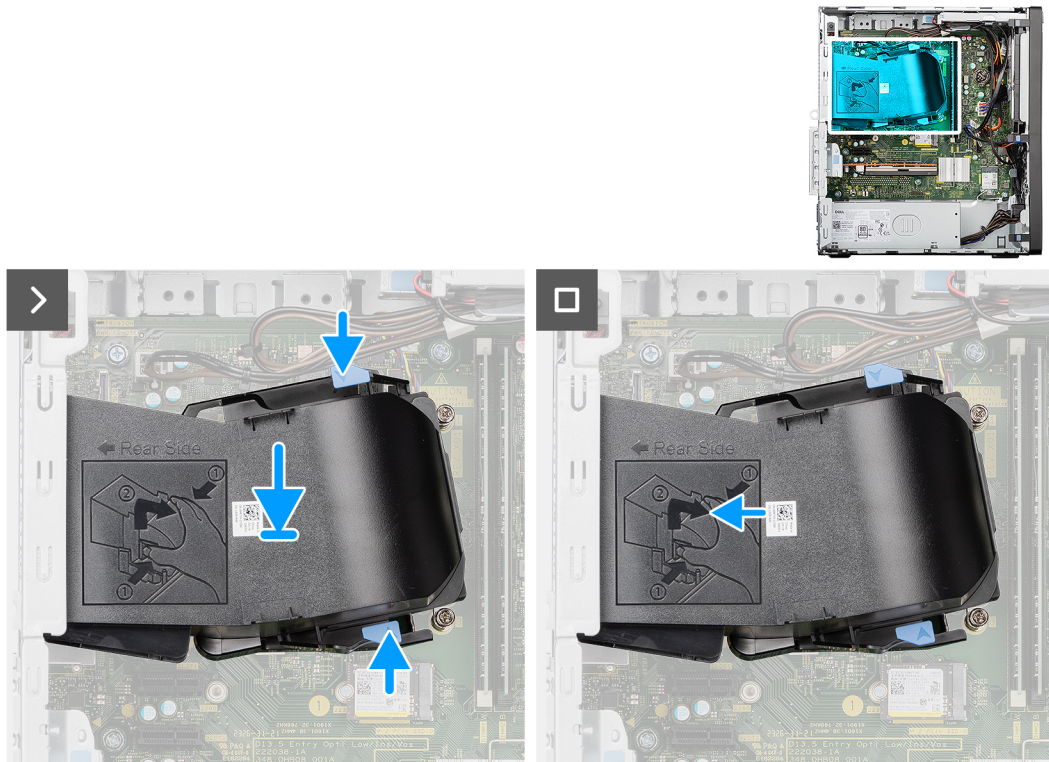
Figura 61. Installazione del condotto della ventola
