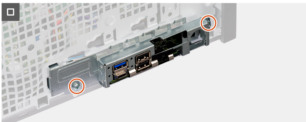
Figura 51. Installazione del pulsante di accensione
