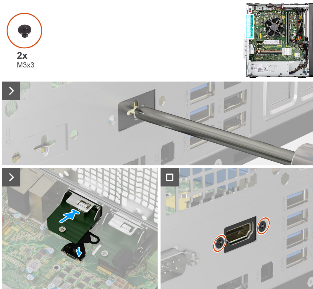
Figura 77. Installare il modulo HDMI opzionale.
