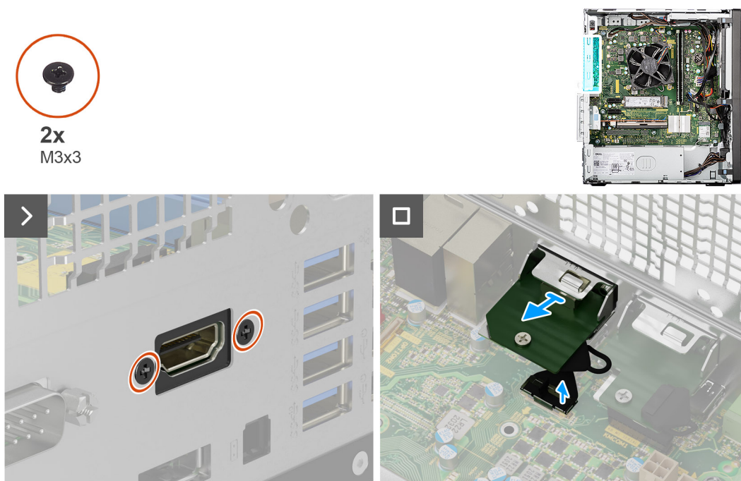
Figura 76. Rimozione del modulo HDMI opzionale
