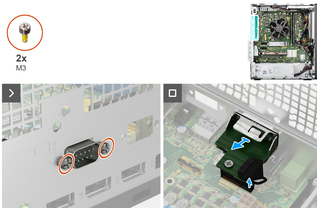
Figura 70. Rimozione del modulo seriale opzionale
