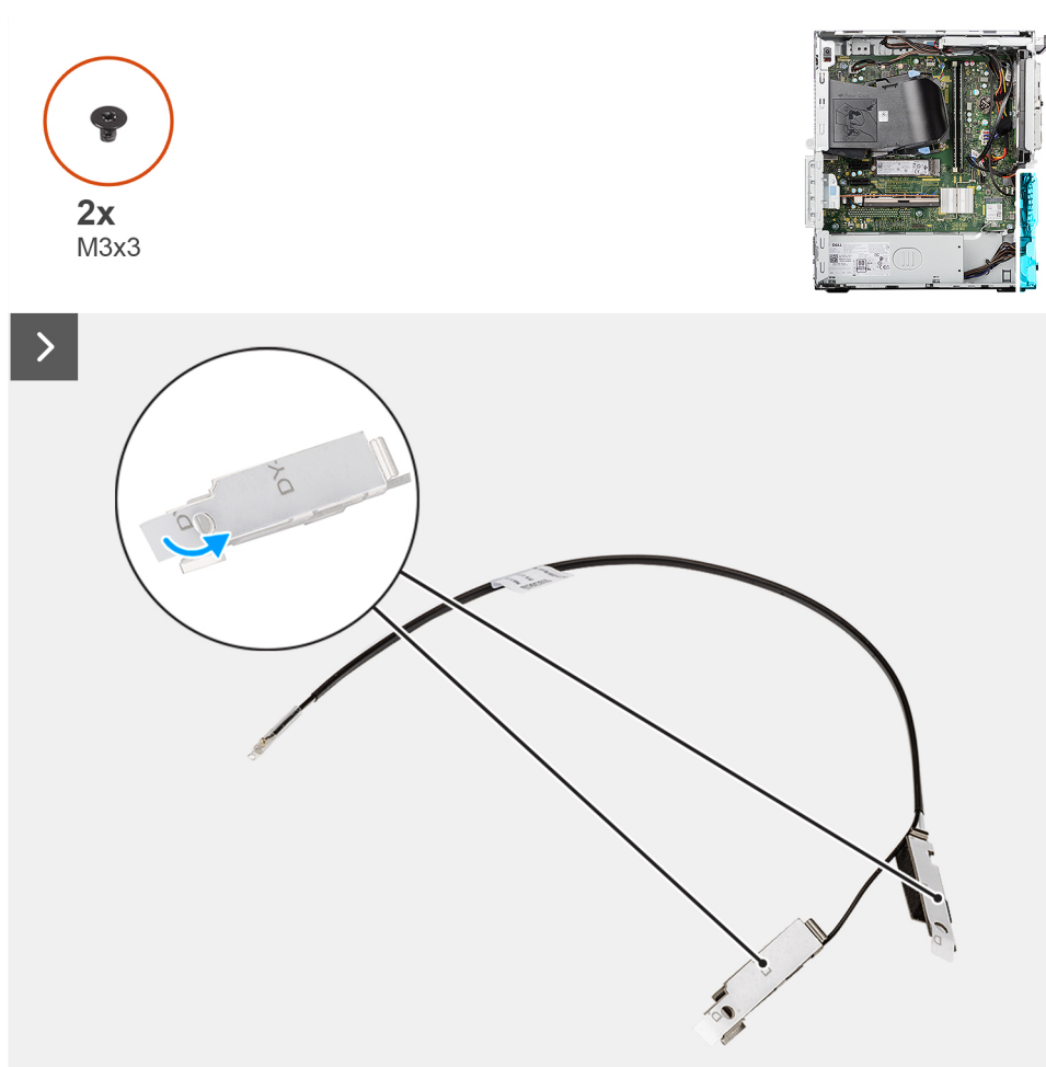
Figura 54. Installazione del modulo dell'antenna interna
