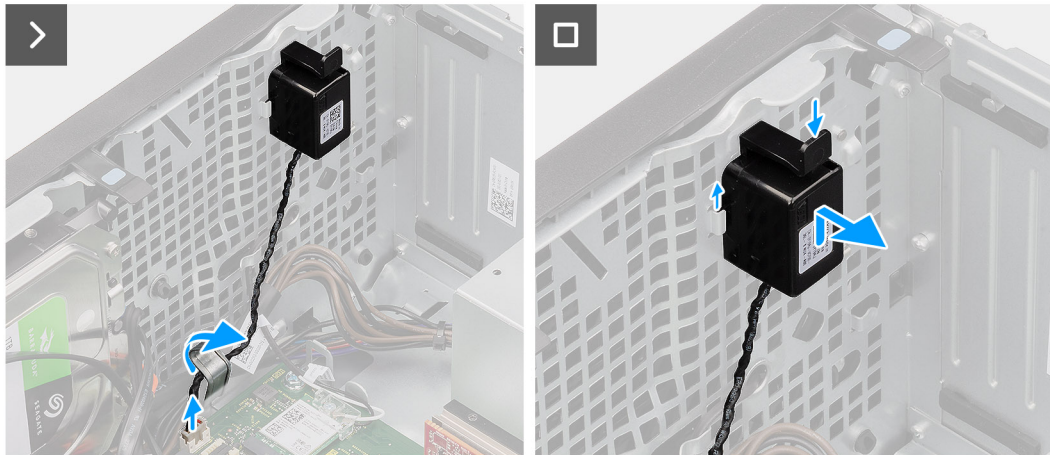
Figura 41. Rimozione dell'altoparlante interno
