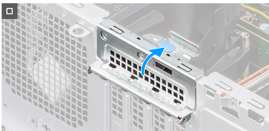
Figura 75. Installazione del modulo seriale e PS2 opzionale
