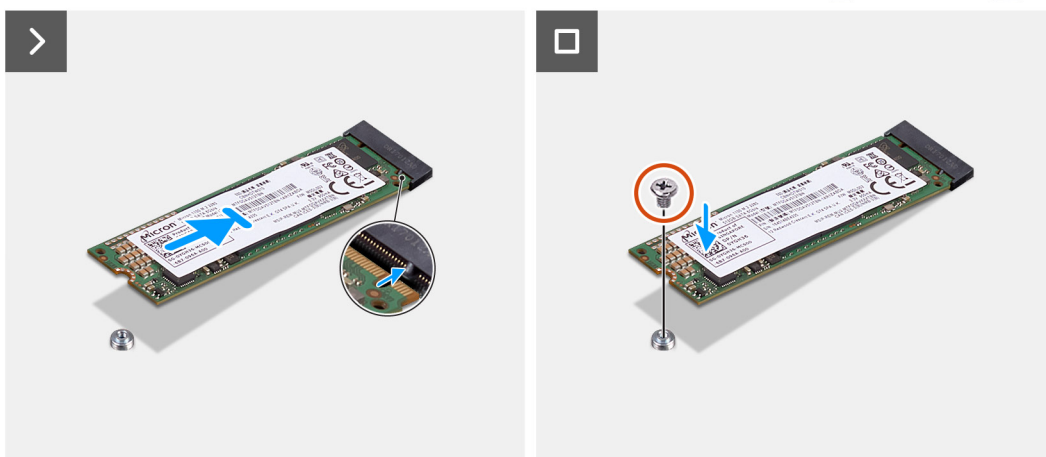
Figura 24. Installazione dell'unità SSD M.2 2280
