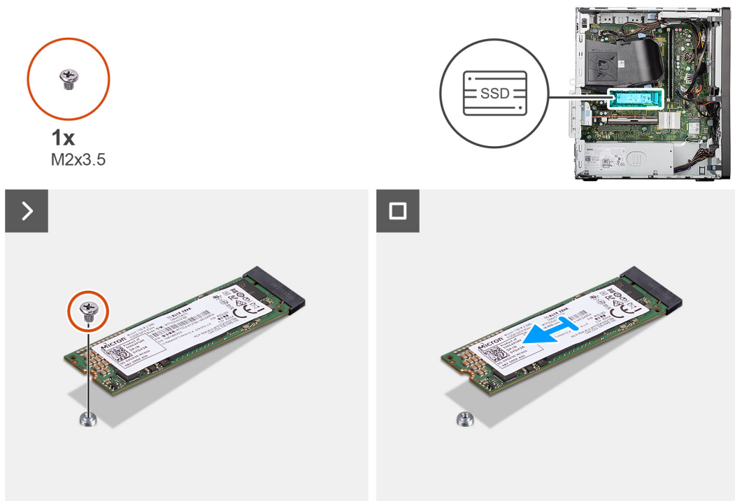
Figura 22. Rimozione dell'unità SSD M.2 2280
