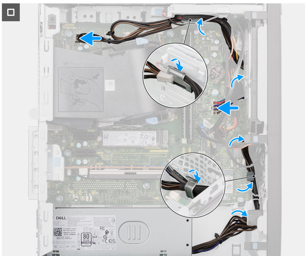
Figura 67. Installazione dell'unità di alimentazione
