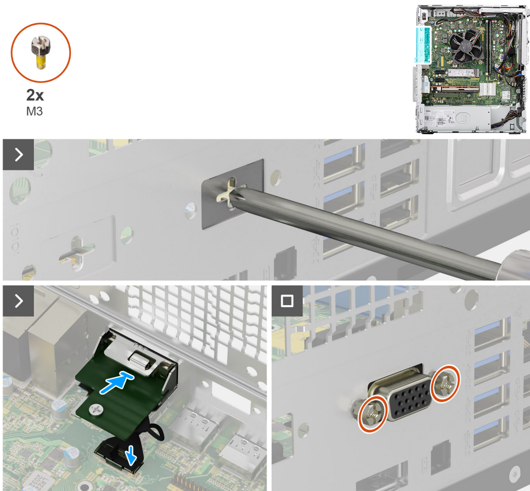
Figura 81. Installare il modulo VGA opzionale.
