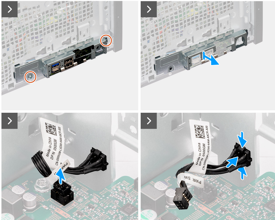
Figura 49. Rimozione del pulsante di accensione
