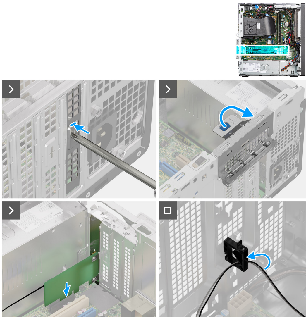
Figura 58. Installazione del modulo dell'antenna SMA esterna
