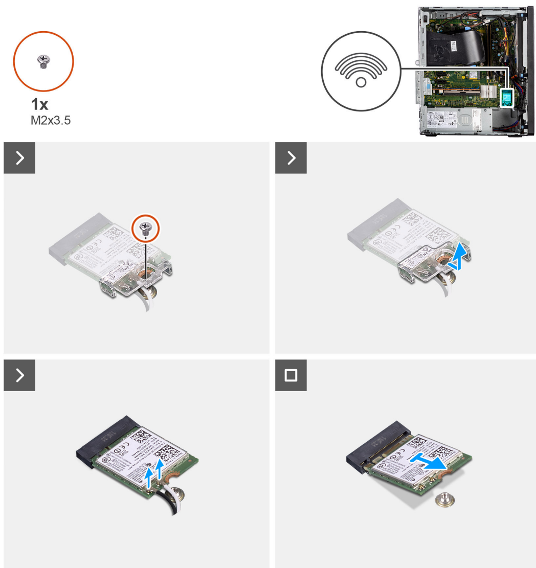
Figura 31. Rimozione della scheda wireless
