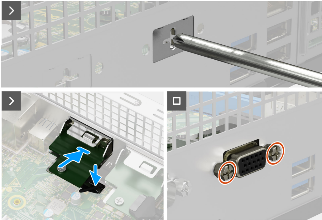
Figura 51. Installazione del modulo VGA
