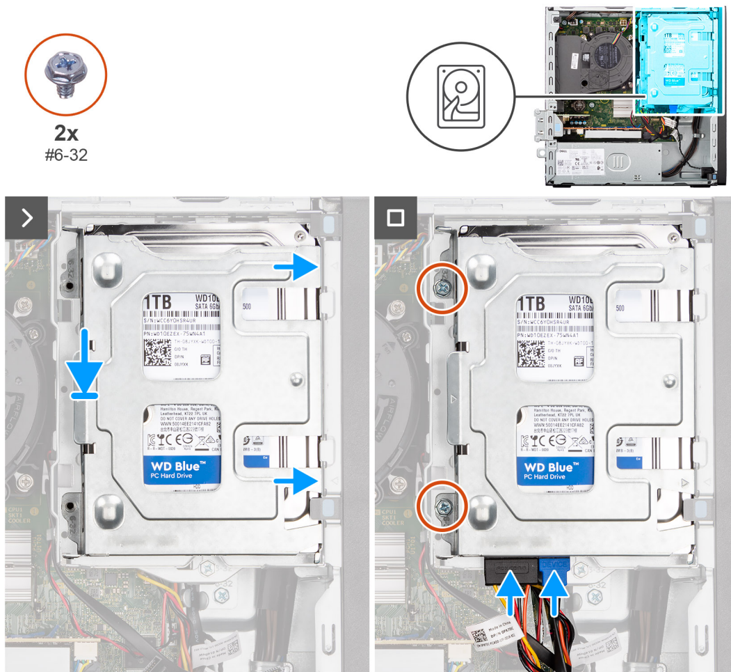
Figura 10. Installazione del disco rigido da 3,5 pollici
