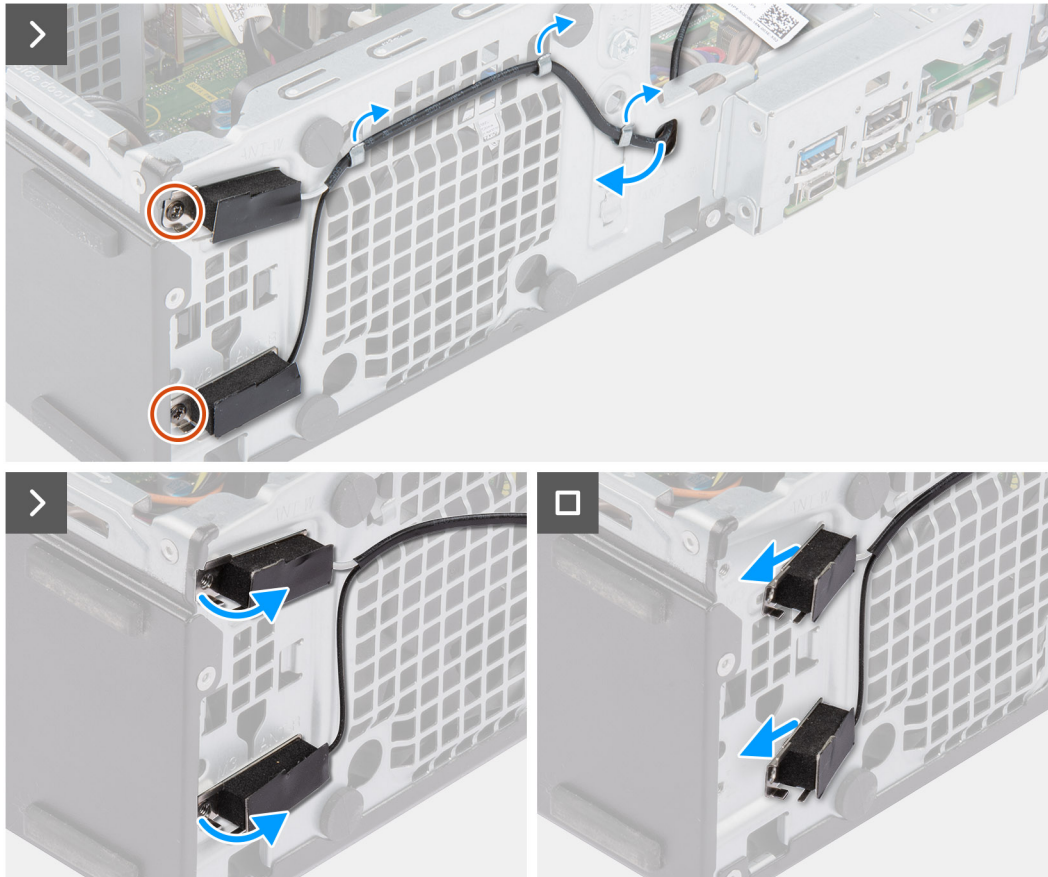
Figura 37. Rimozione del modulo dell'antenna interna
