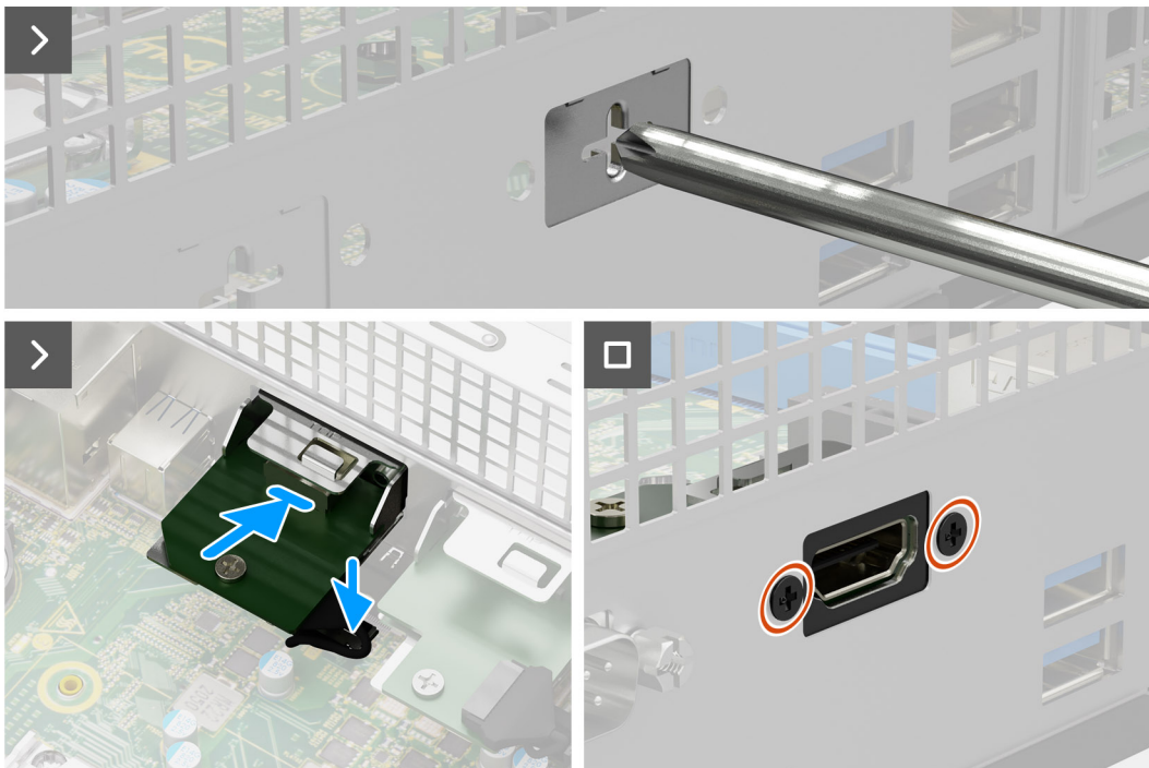
Figura 55. Installazione del modulo HDMI
