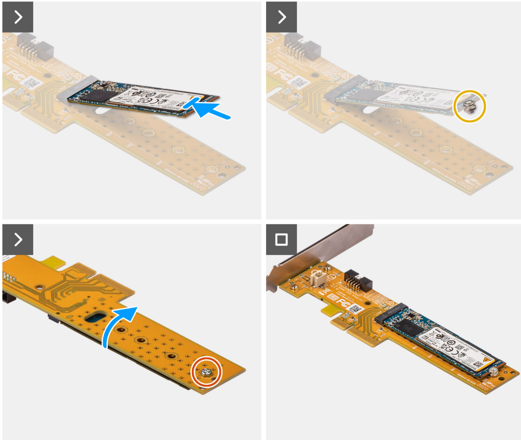
Figura 25. Installazione dell'unità SSD M.2 2280 sulla scheda Dell Ultra Speed Drive Gen3
