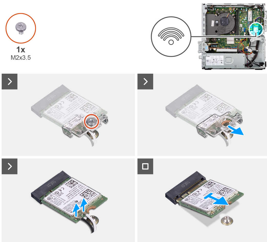
Figura 27. Rimozione della scheda wireless
