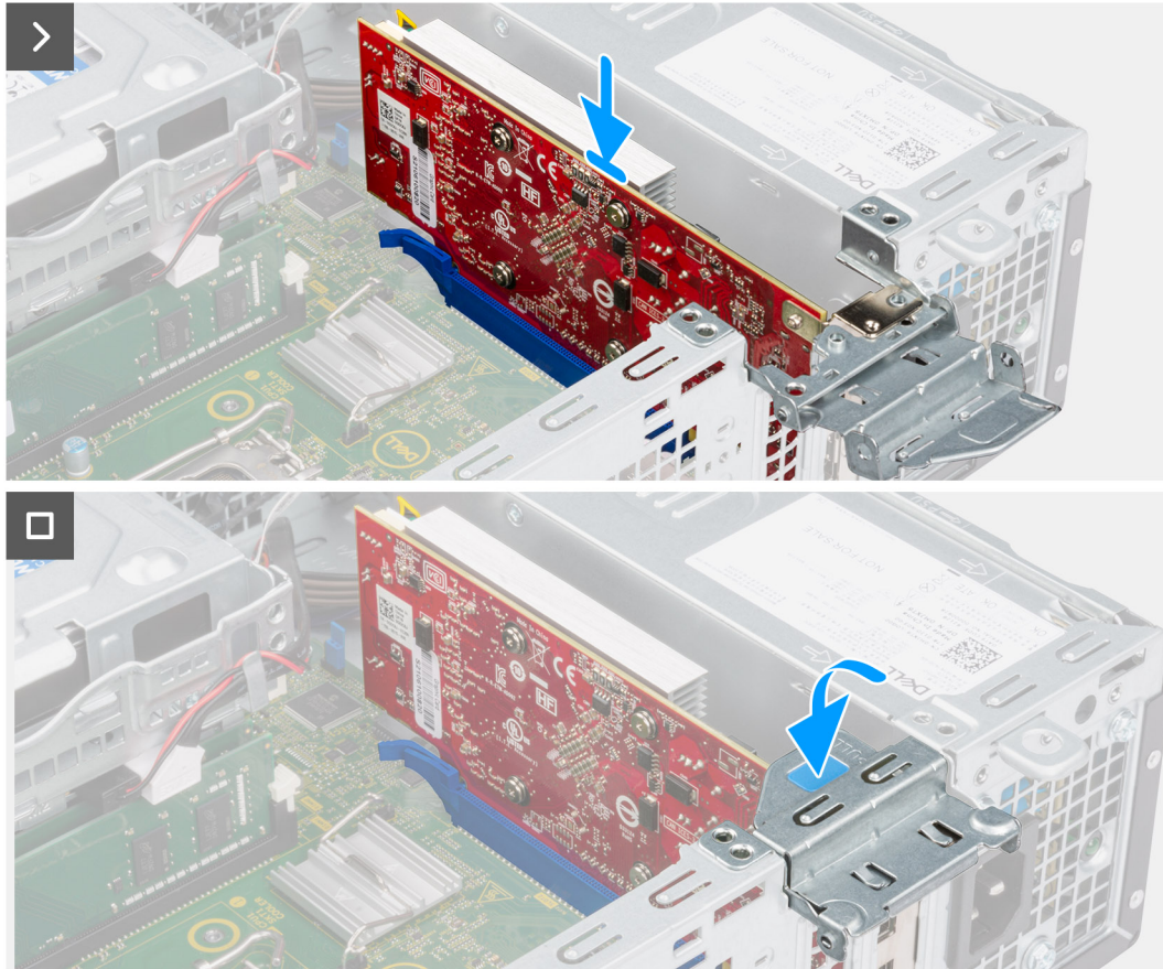
Figura 30. Installazione della scheda grafica
