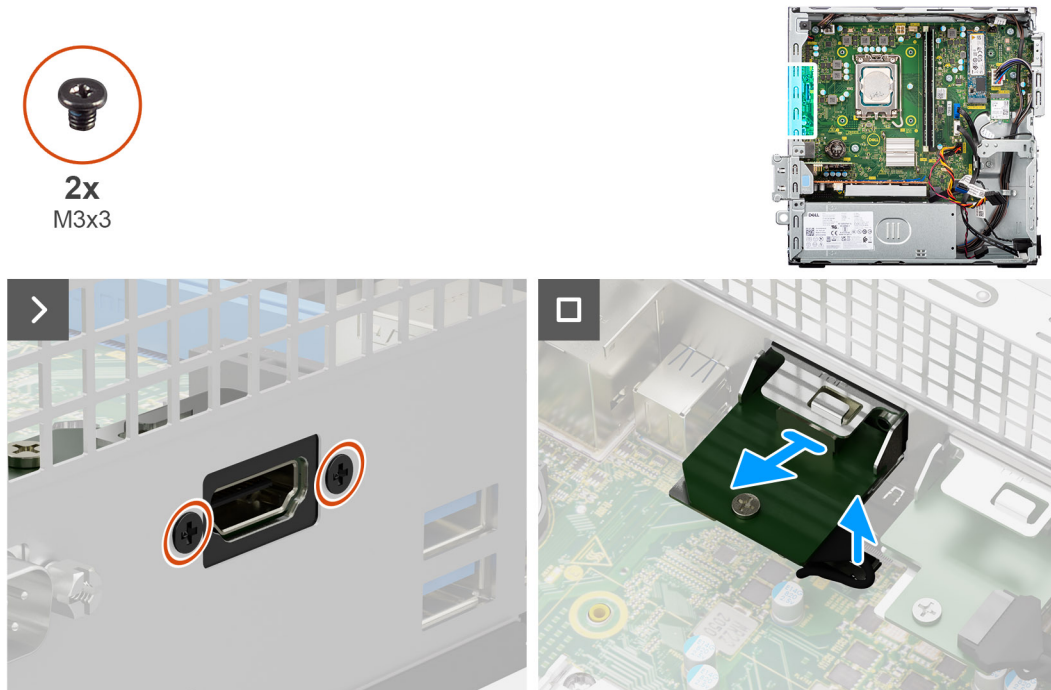
Figura 54. Rimozione del modulo HDMI
