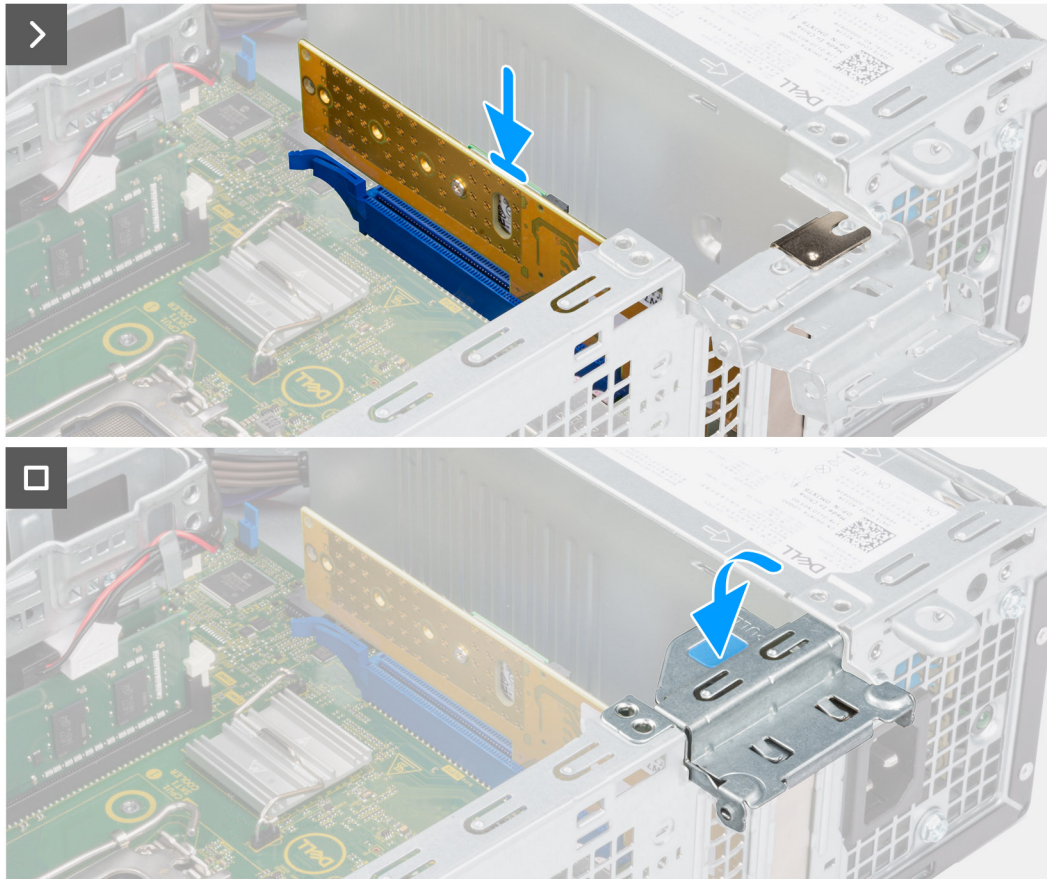
Figura 26. Installazione della scheda Dell Ultra Speed Drive Gen3
