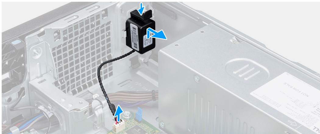
Figura 31. Rimozione degli altoparlanti
