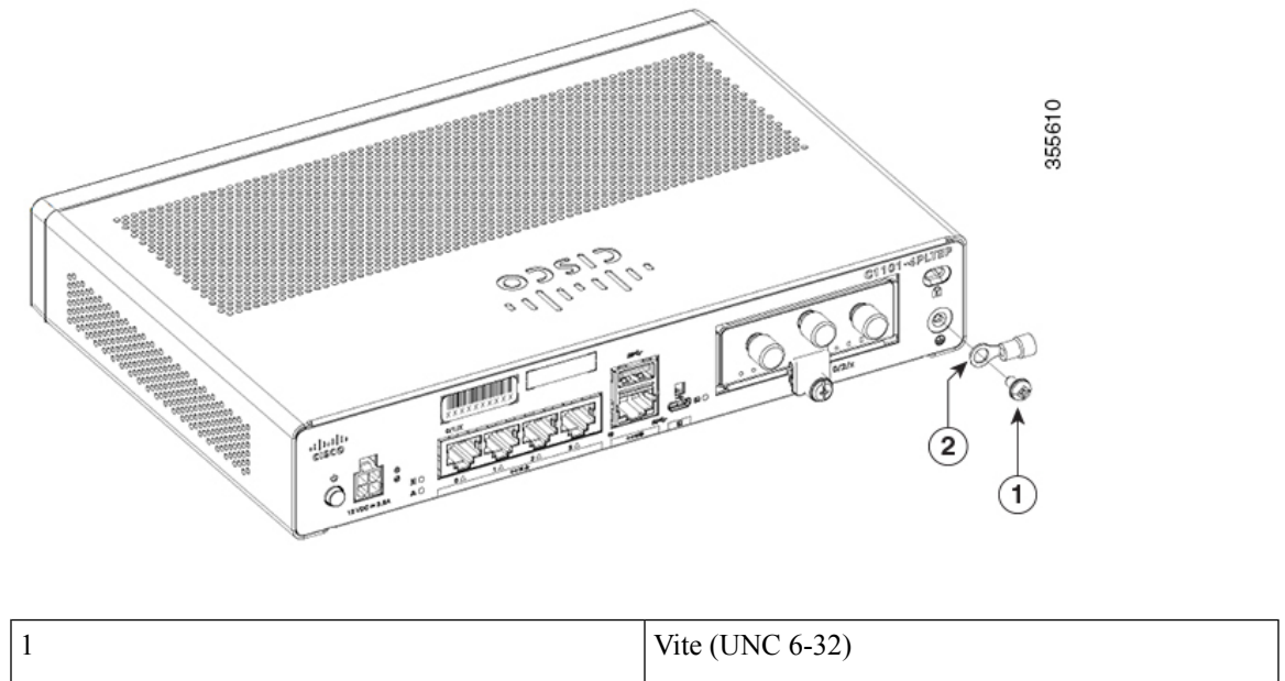
Figura 48: Messa a terra dello chassis - Cisco 1101-4PLTEP
